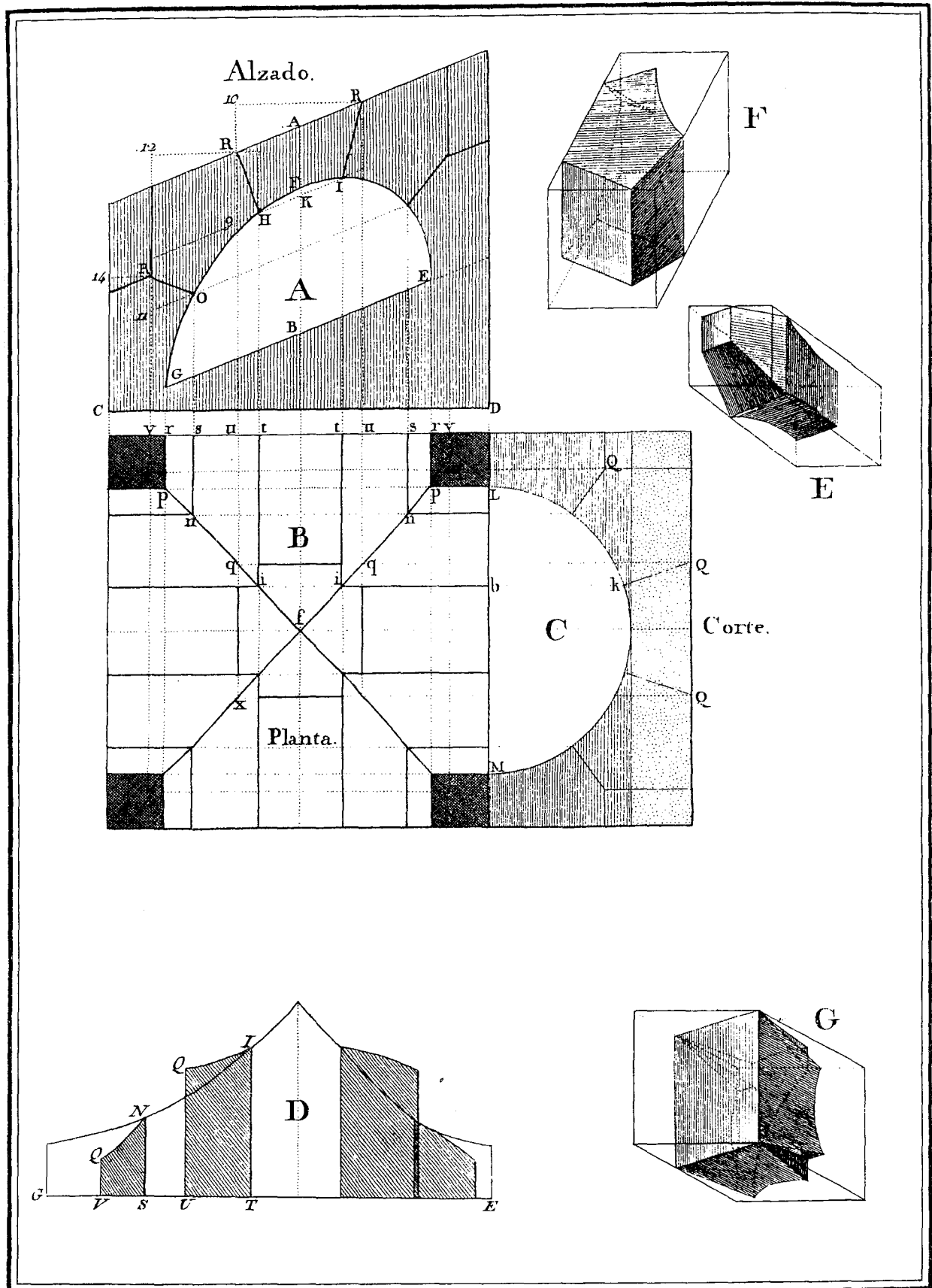
BOVEDA POR ARISTA FORMADA POR UN ARCO EN rampa en una bajada.
