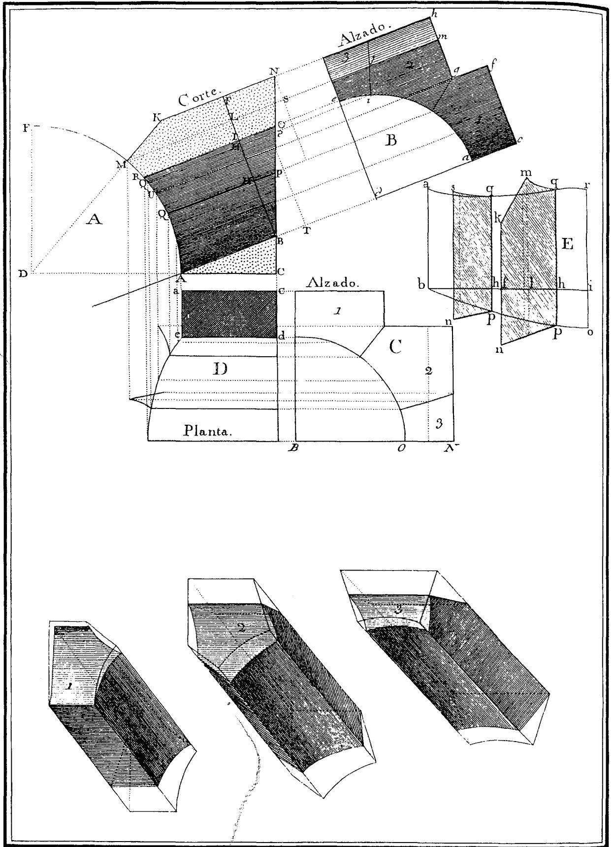
LUNETTO DESCENDENTE.
