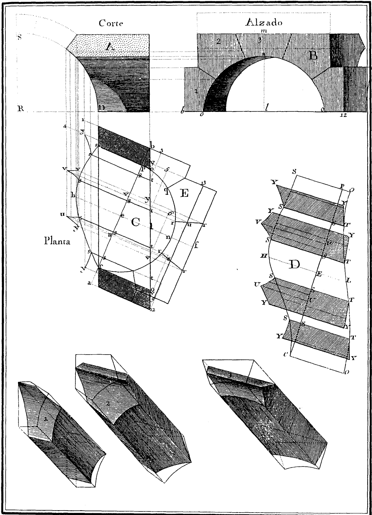
LUNETO OBLIQUO. 2
