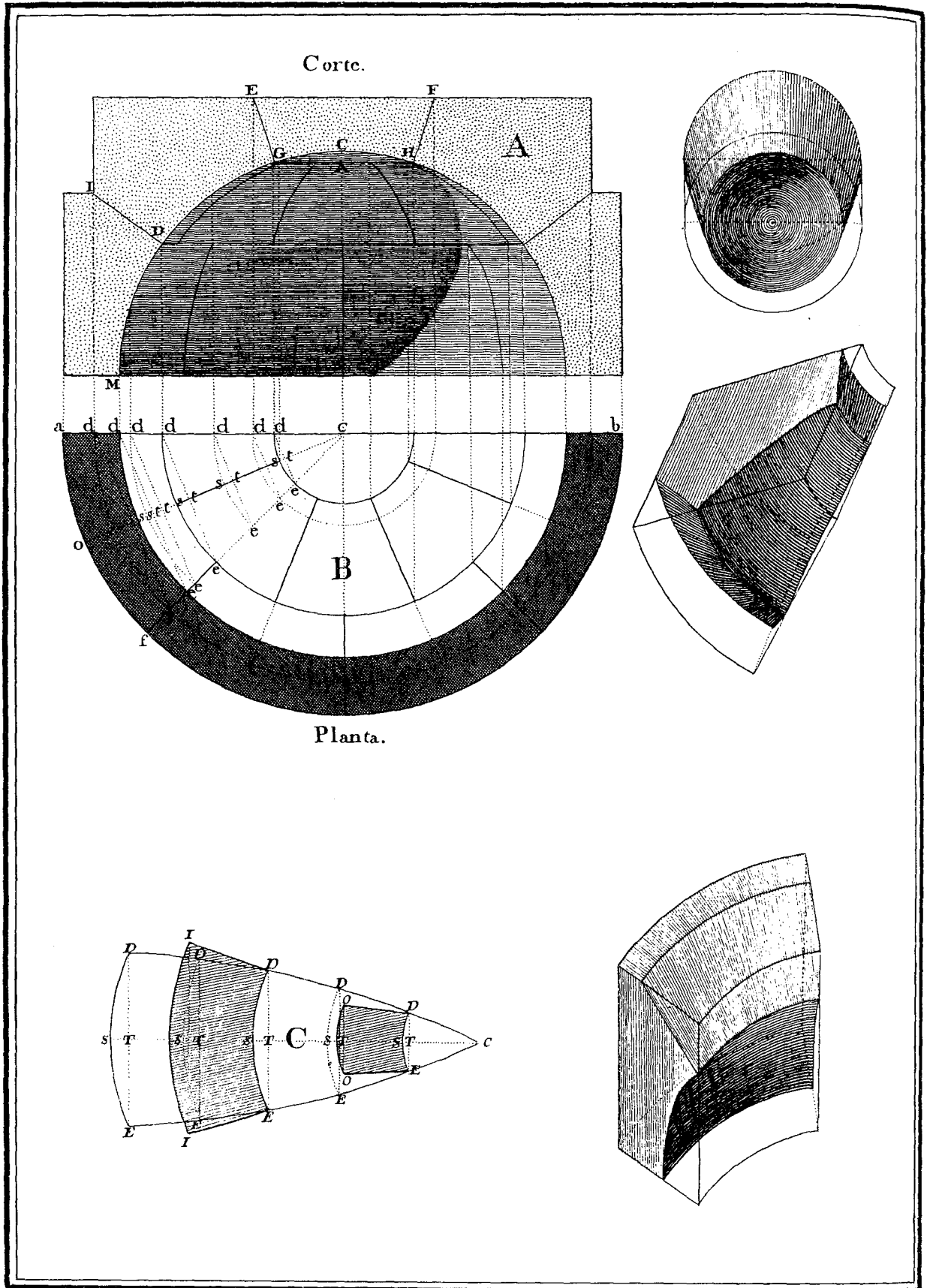
BOVEDA ESFERICA.
