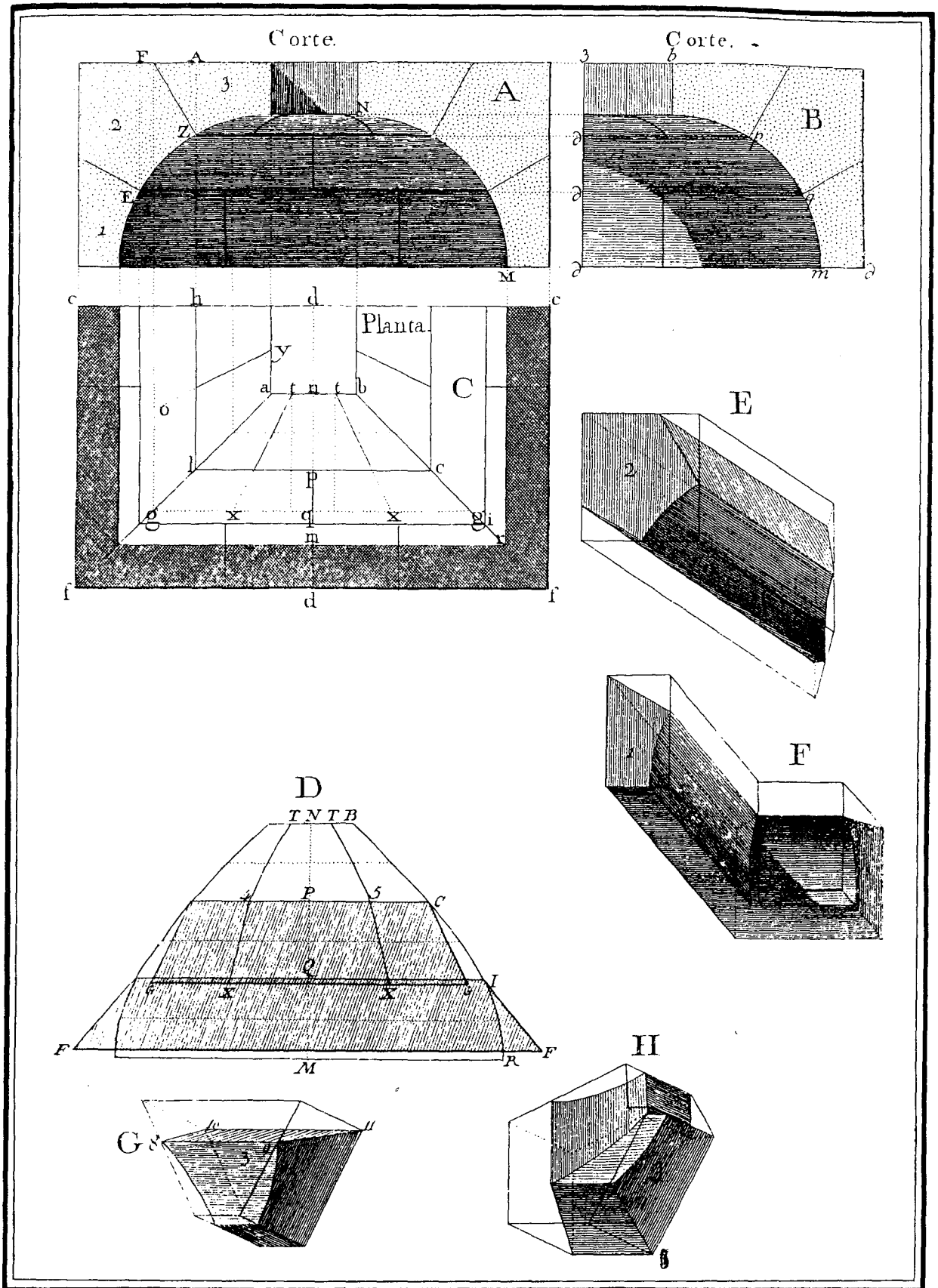
BOVEDA EN RINCON DE CLAUSTRO CON CLARABOYA y de Planta quadrilonga.
