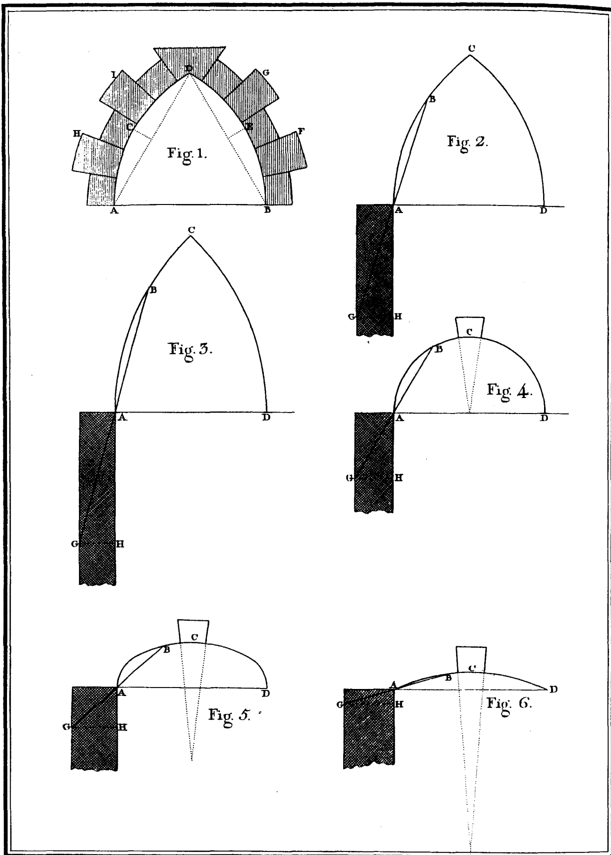
CORRESPONDENCIA DE LOS ESTRIVOS CON respecto á la curvâ de la Boveda.
