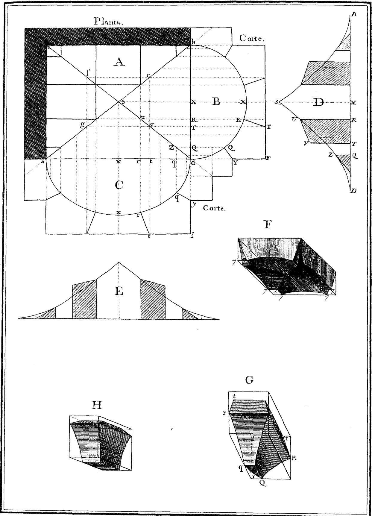
BOVEDA POR ARISTA SOBRE UN QUADRILONGO.
