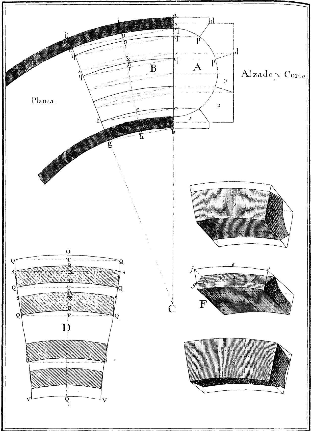
CAÑON DE BOVEDA CIRCULAR.
