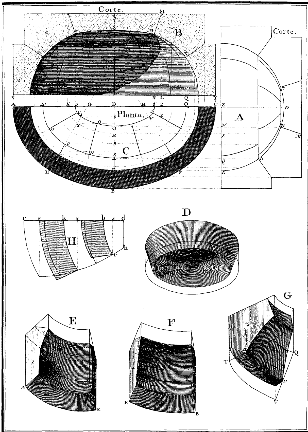
BOVEDA ELIPTICA.
