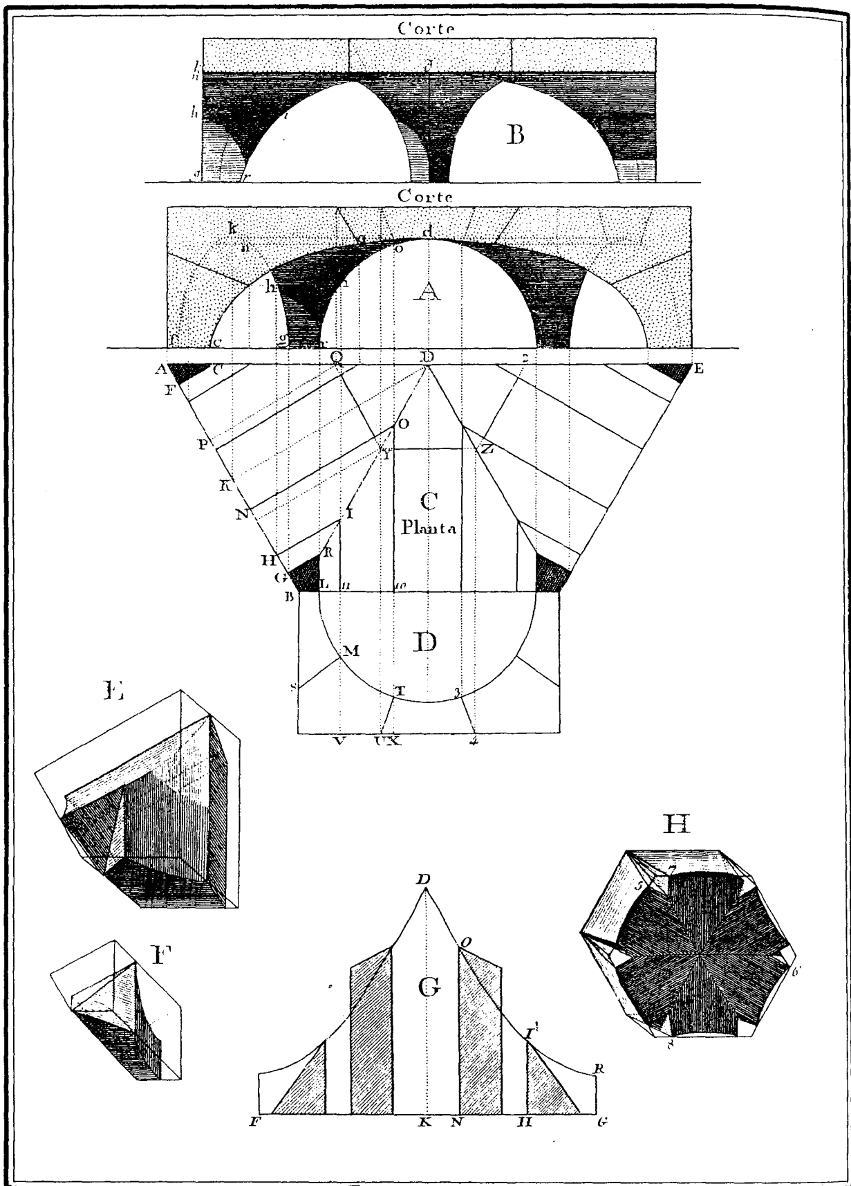
BOVEDA POR ARISTA SOBRE UN EXAGONO.
