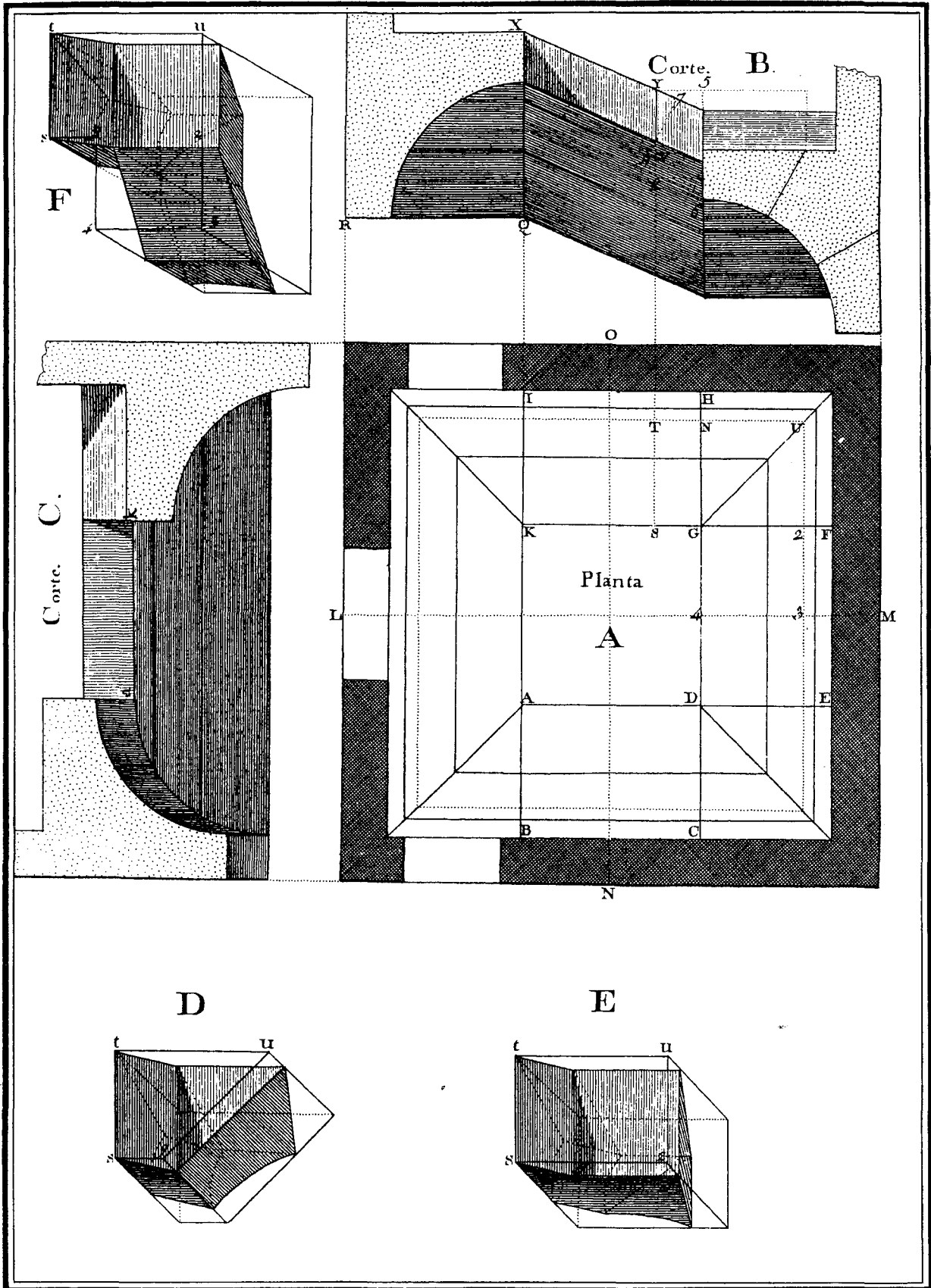
ESCALERA EN SEMI-CANÓN SUSPENDIDO.
