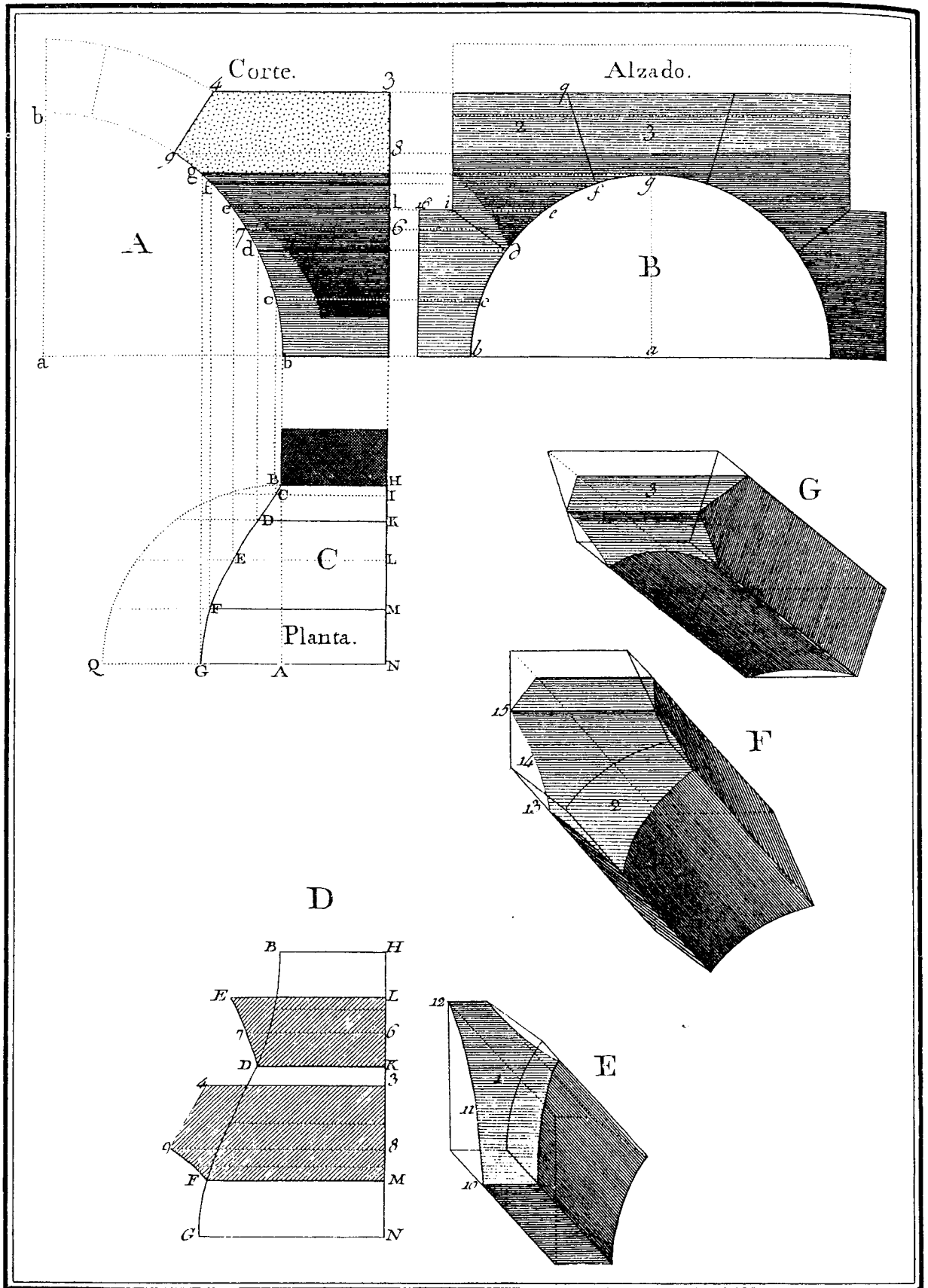
LUNETO RECTO.
