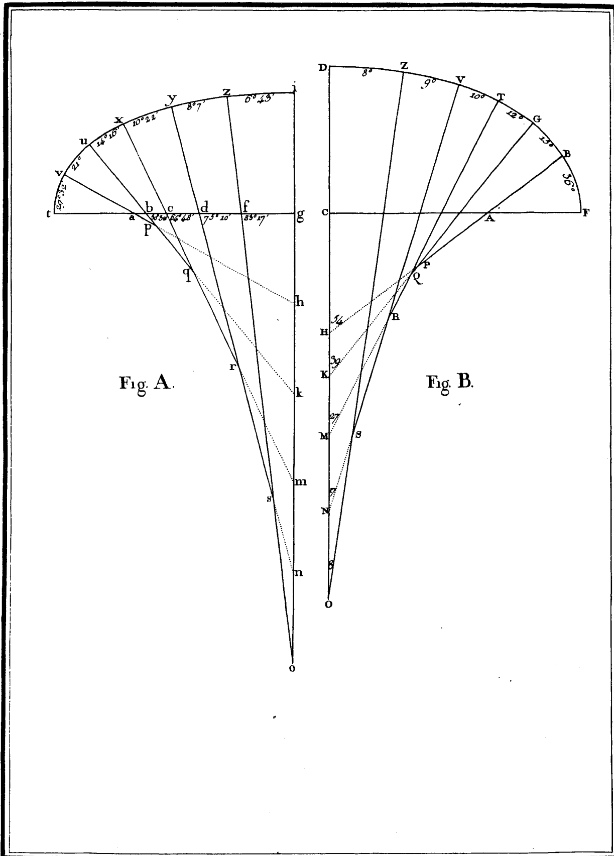
BOVEDA DE ONCE CENTROS EN DOS SUPOSICIONES diferentes.
